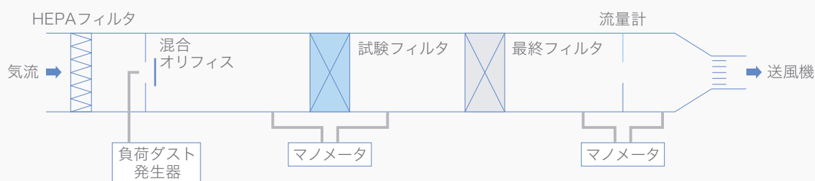
質量法捕集率を求める試験装置の概略図
