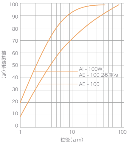
AI・AE 粒径別捕集効率 (標準風速時)
