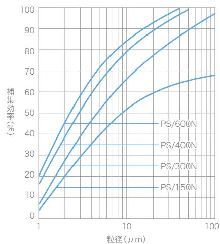
PS 粒径別補集効率(標準風速時)
