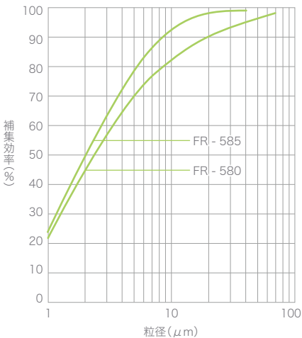
FR 粒径別補集効率(標準風速時)
