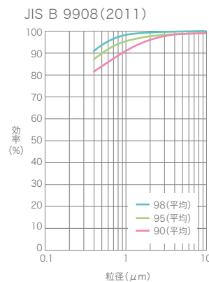
粒径別捕集率の関係
