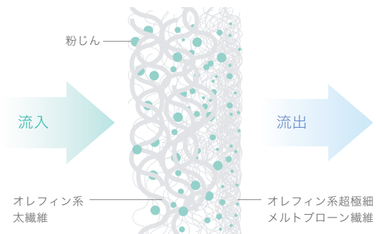
連続密度勾配ろ材
