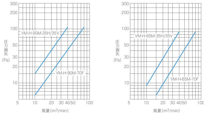
風量と圧力損失の関係
